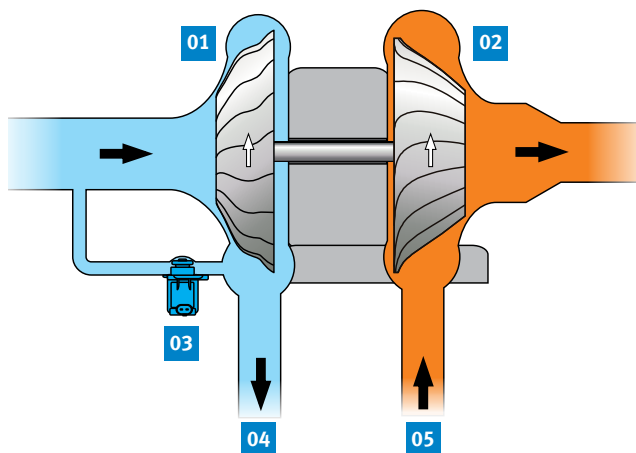
Funzionamento di una valvola di ricircolo dell'aria in fase di rilascio:
